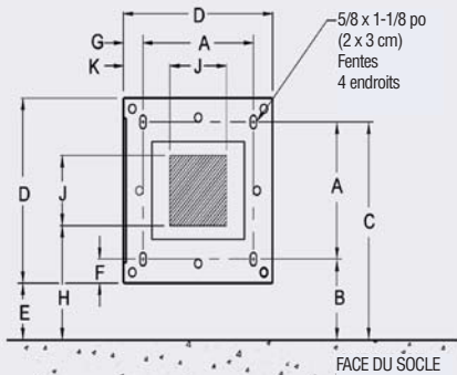
EMPLACEMENT DES BOULONS
