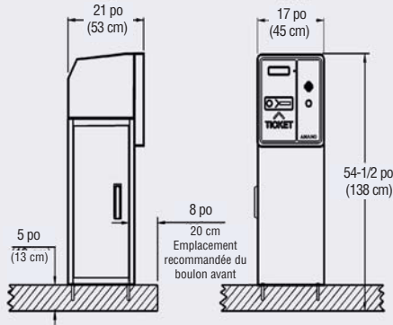
EMPLACEMENT DES BOULONS
